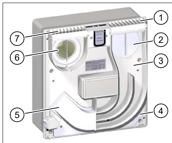
Obr. 6: Větrací jednotka – sejmuté víko jednotky
