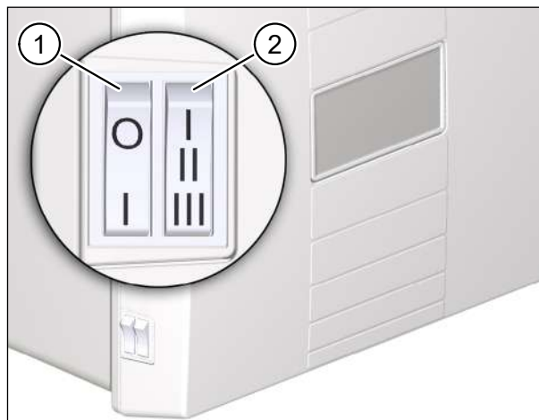
Obr. 10: Ovládací prvky na větrací jednotce
