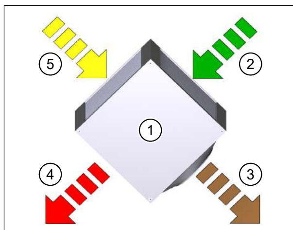
Obr. 9: Princip fungování deskového výměníku tepla s křížovým tokem
