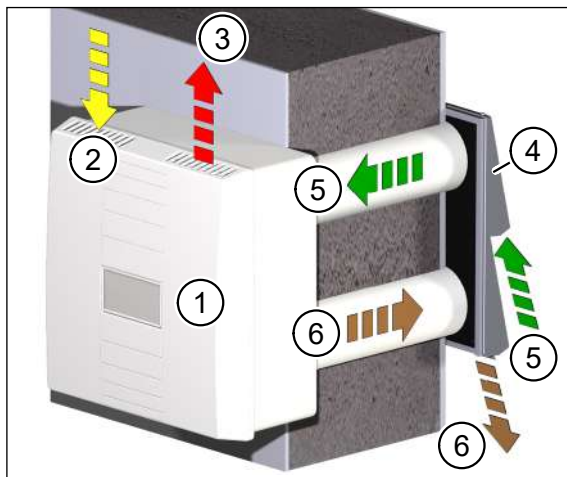
Obr. 7: Princip fungování větrací jednotky
