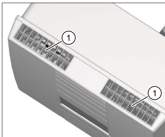
Obr. 12: Otevřené vzduchové klapky
