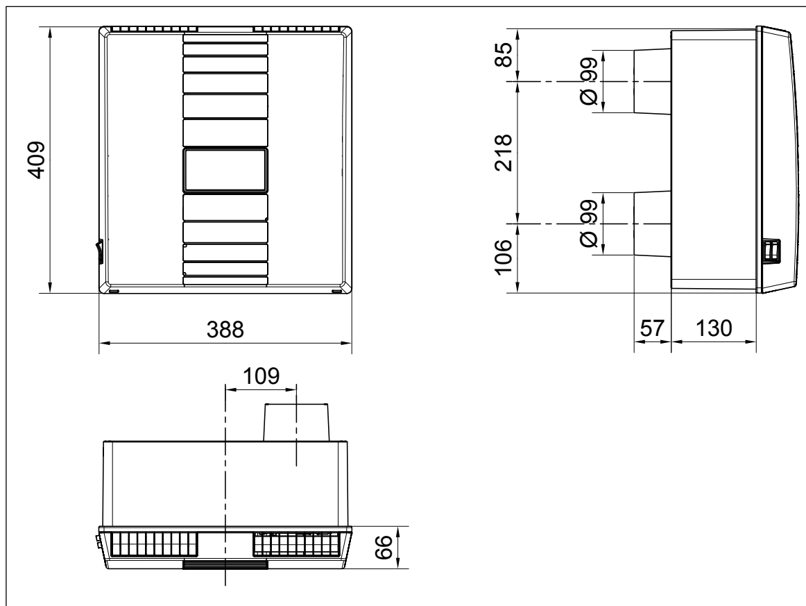
Obr. 4: Rozměry větrací jednotky M-WRG-S v mm
