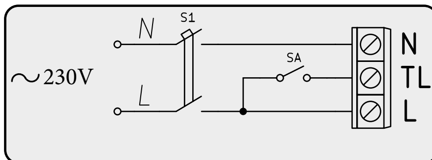
Elektrické schéma pro připojení ventilátorů s možností časovače.
